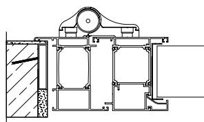
APPLICAZIONE A "Z"
