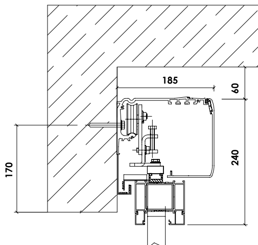
APPLICAZIONE SU MURATURA
