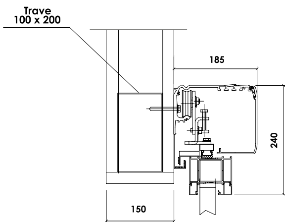
APPLICAZIONE SU TRAVE IN CTG
